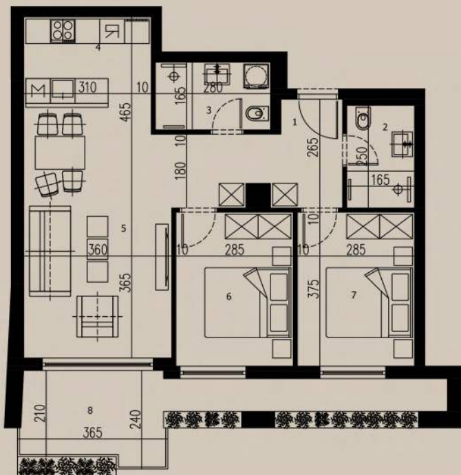
OSNOVA STANA
