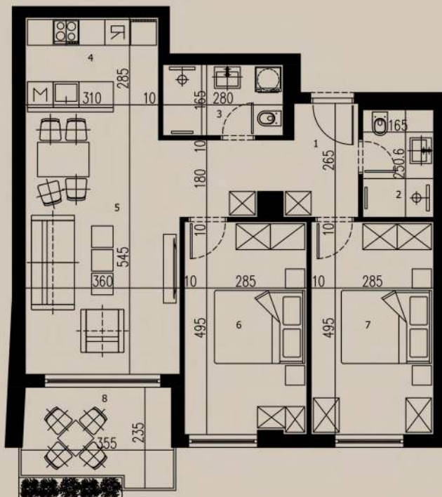
OSNOVA STANA
