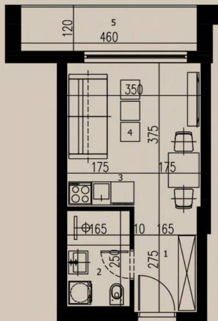
OSNOVA STANA
