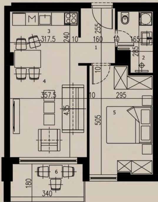
OSNOVA STANA
