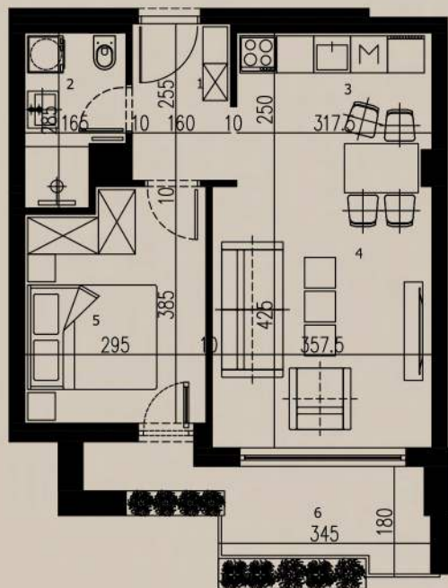
OSNOVA STANA
