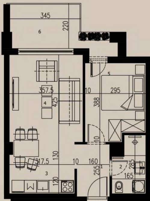
OSNOVA STANA
