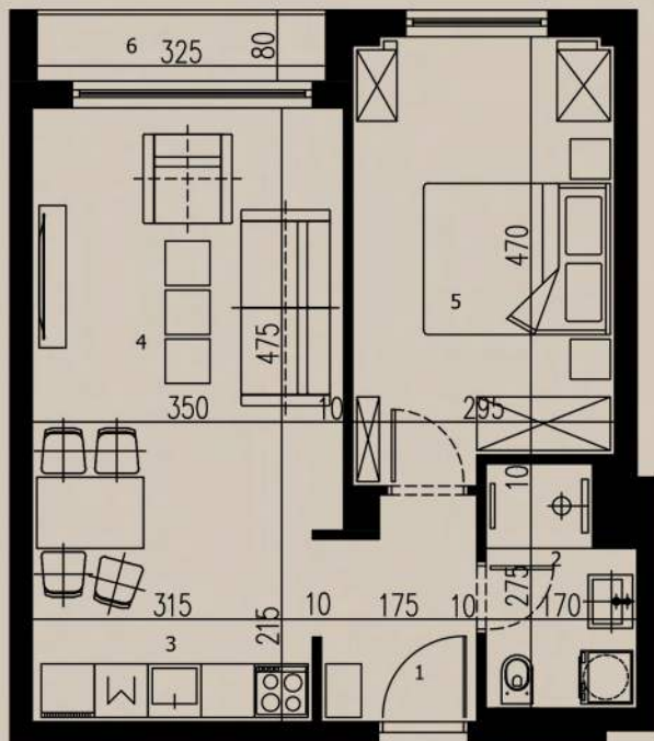
OSNOVA STANA
