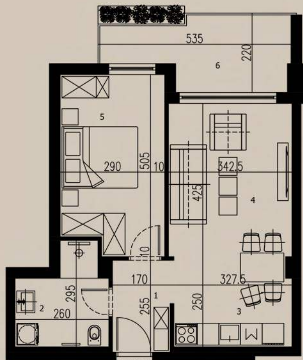
OSNOVA STANA
