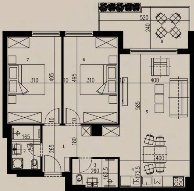
OSNOVA STANA
