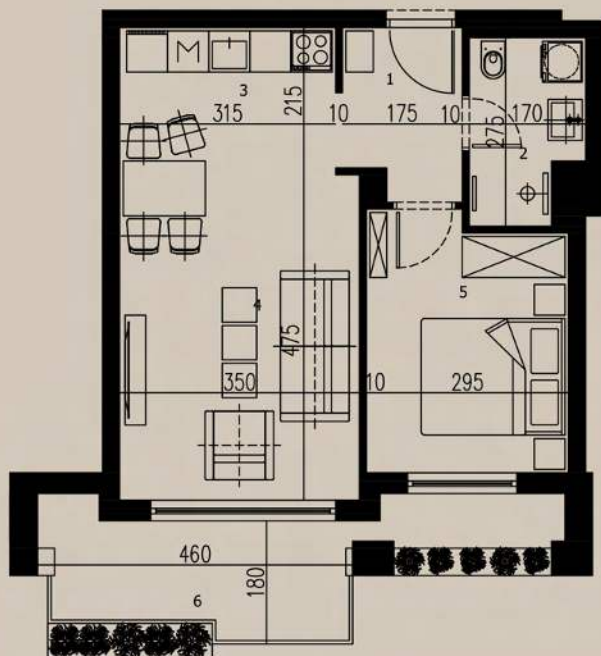
OSNOVA STANA
