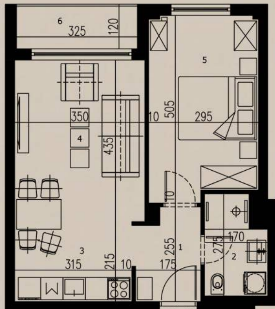
OSNOVA STANA
