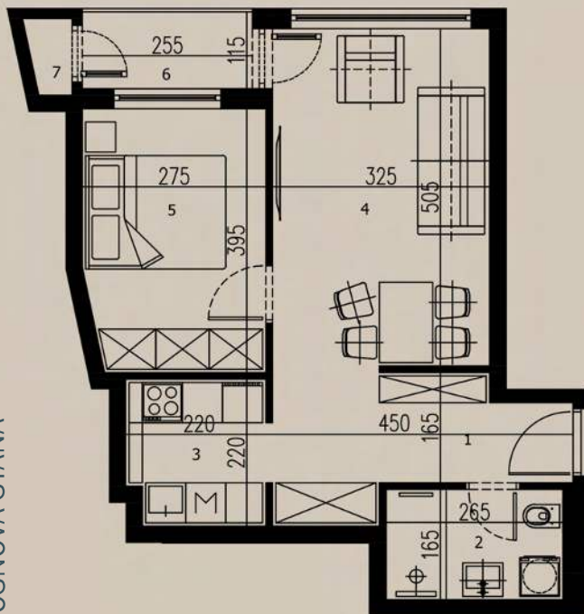
OSNOVA STANA
