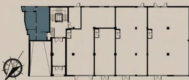
OSNOVA SPRATA
